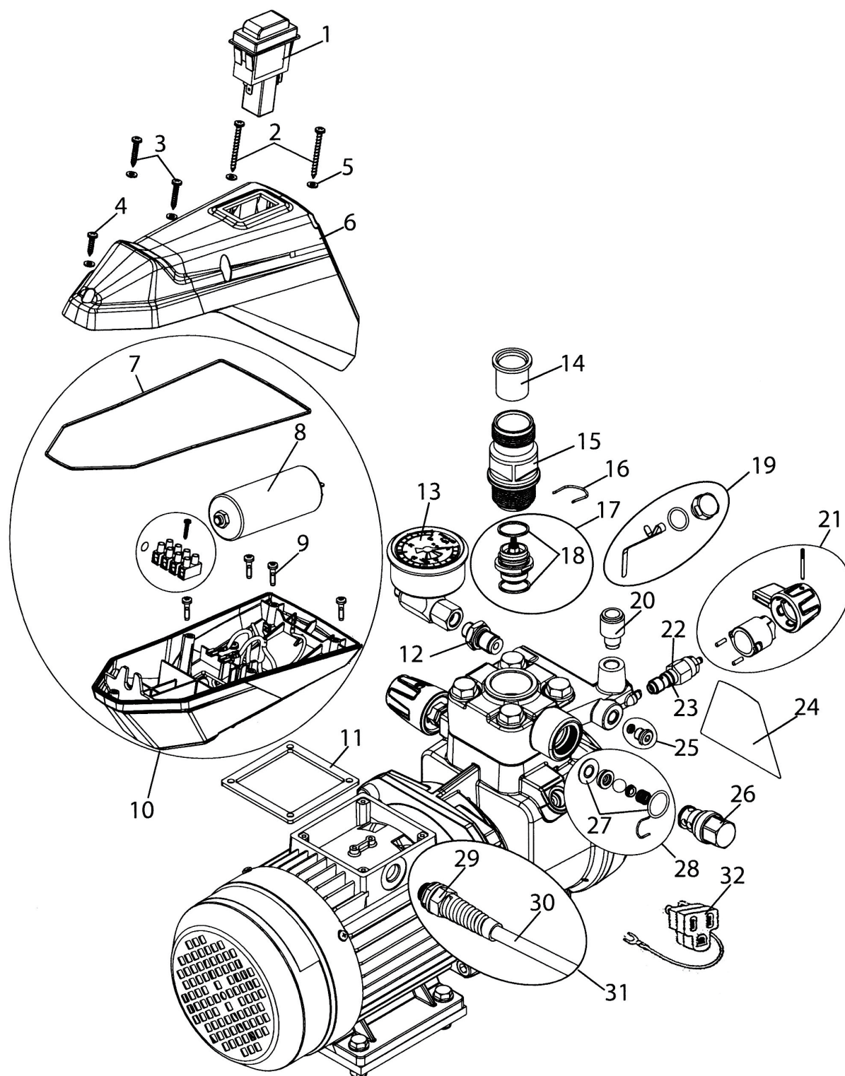
HERO23 motor
